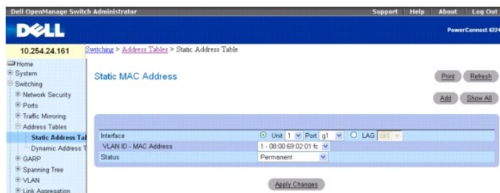
Ilustración 8-32. Dirección MAC estática
